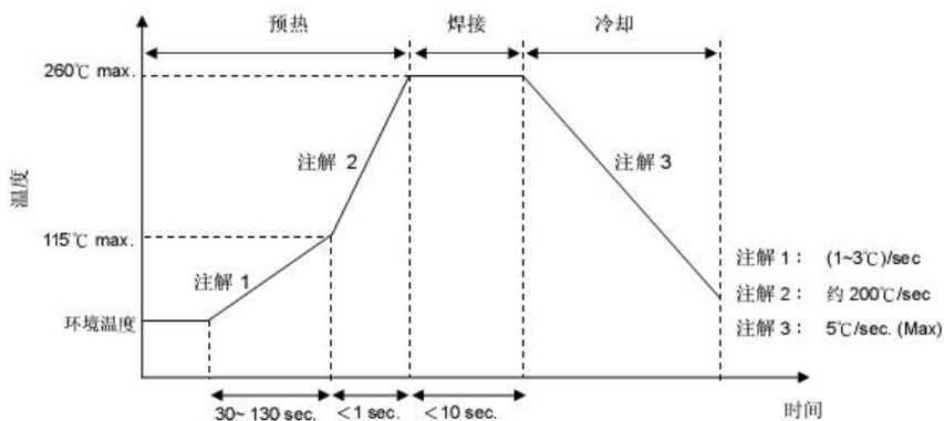
波峰焊曲线
